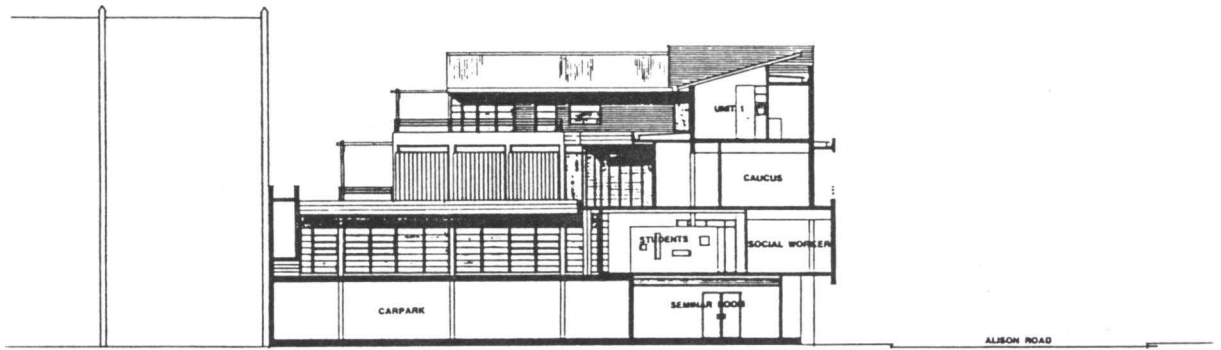
SECTION A-A SCALE 1:100
