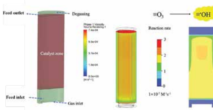
图1. 化学动力学-计算流体力学对催化臭氧过程的典型模拟结果
